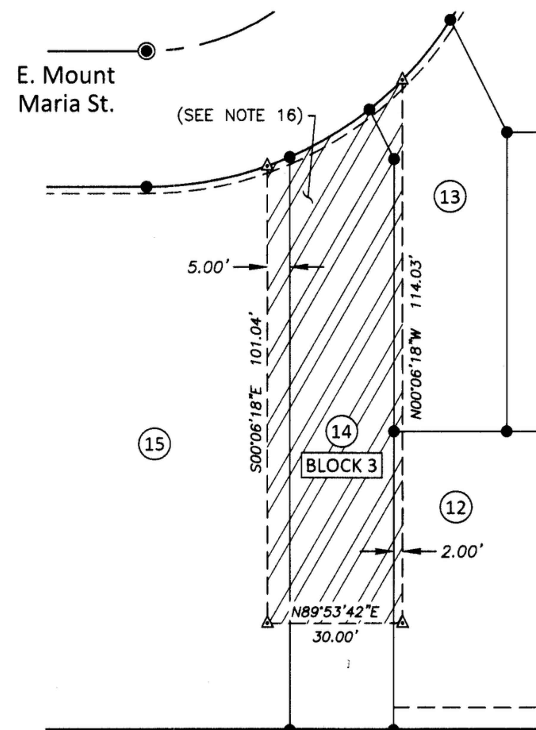
DETAIL "C" SCALE: 1"=30'
